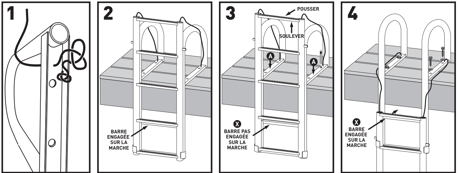
Fig. 2 Échelle à la position de repos.
